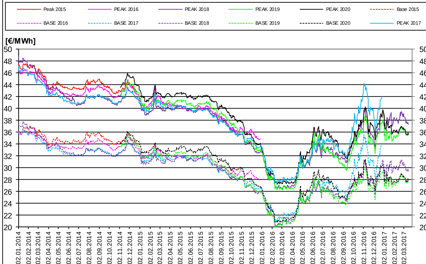
EEX Forward Price Evolution depuis le 01.01.2014
